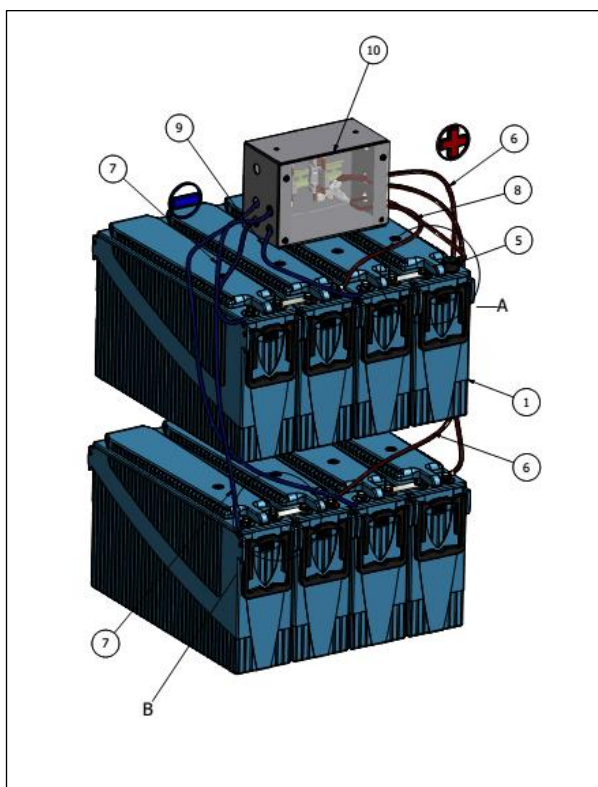
Fig.4: Cablaggi RES 24 x 4
