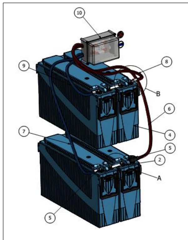
Fig.9: Cablaggi RES 24 x 2
