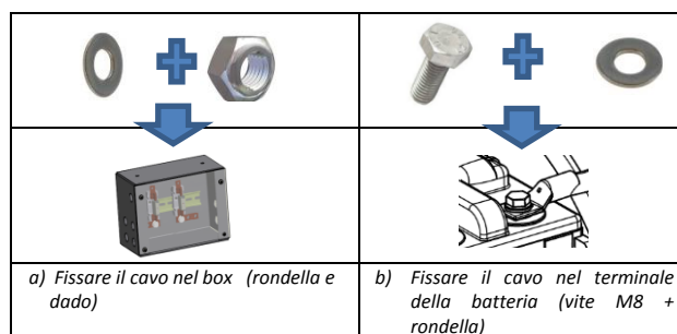
Fig. 8: Fissaggio cavi.
