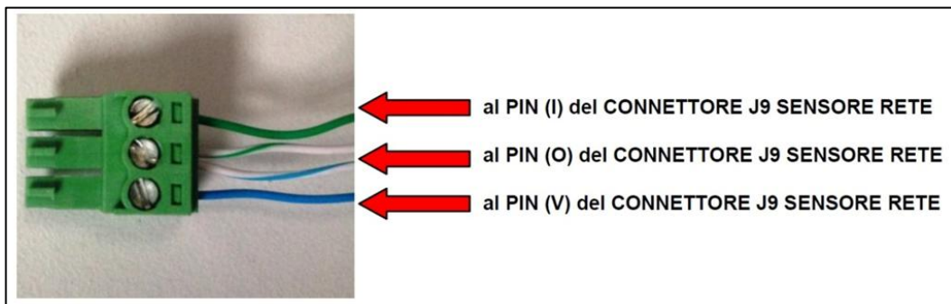
Figura 5 – Cablaggio connettore sensore di rete
