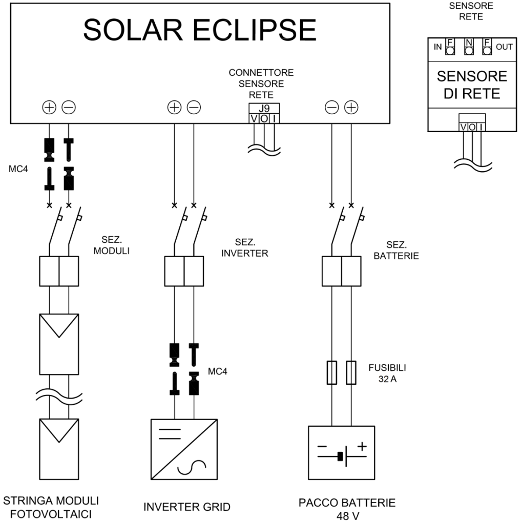
Figura 6 – Schema Cablaggio di potenza
