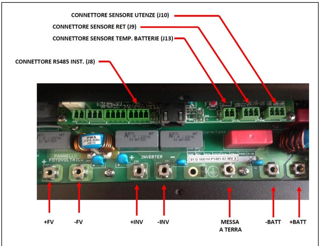
Figura 7 – Cablaggio scheda Solar Eclipse
