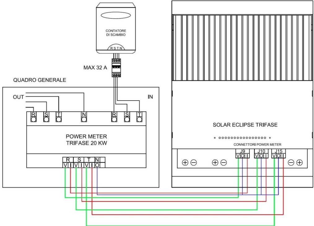
Figura 9 – Cablaggio Power Meter trifase 20 kW
