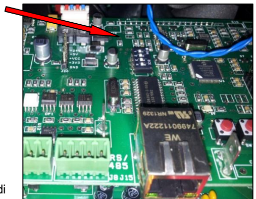
Figura 10 – Dip-Switch di configurazione
