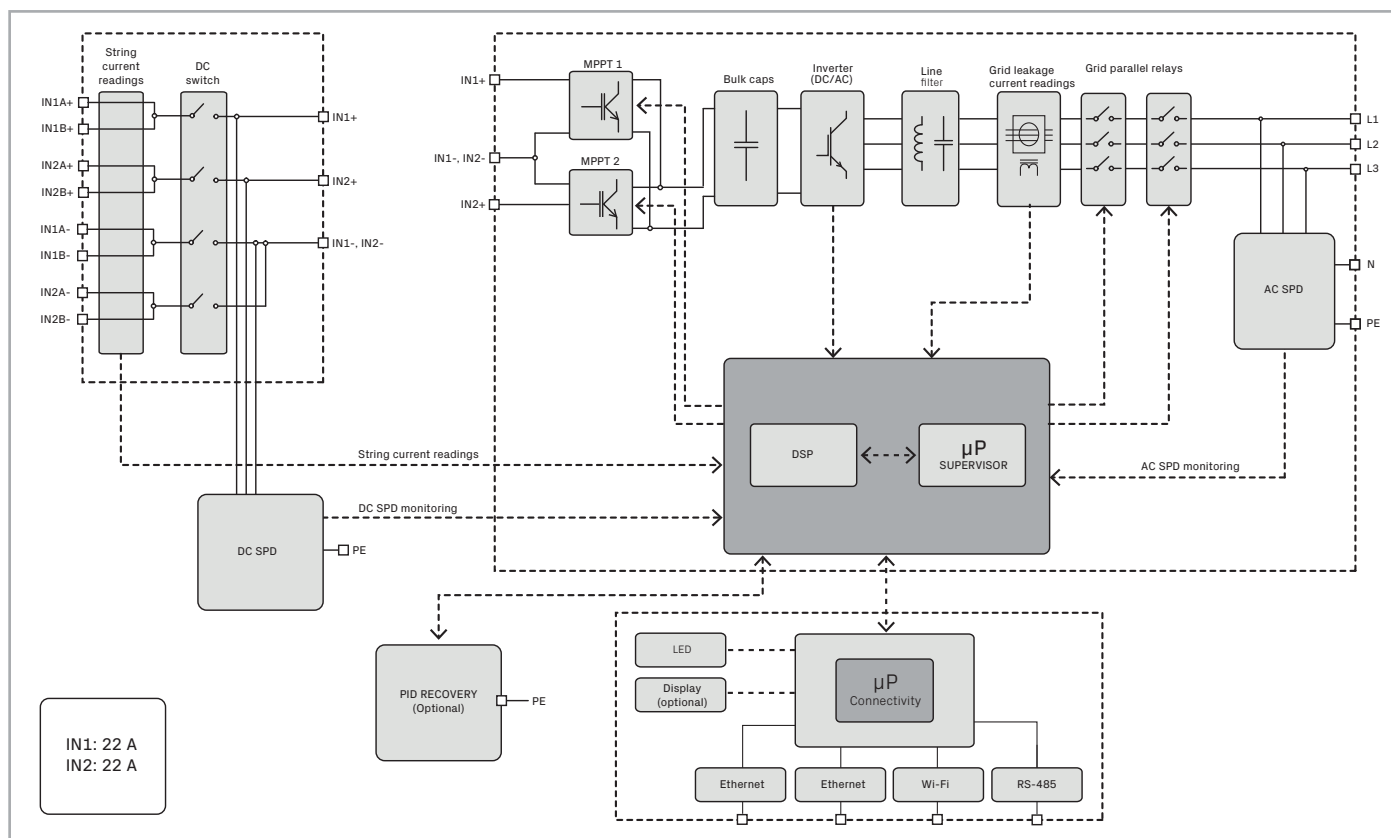
Diagramma a blocchi PVS-10-12.5-15-TL
